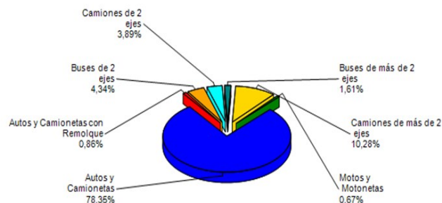
Grafico 2: Distribución de Flujos (transacciones) de Enero, por categoría de vehículo. Fuente : Reporte 29 - SICE
